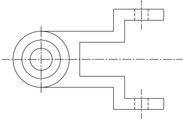
TOP SIDE
